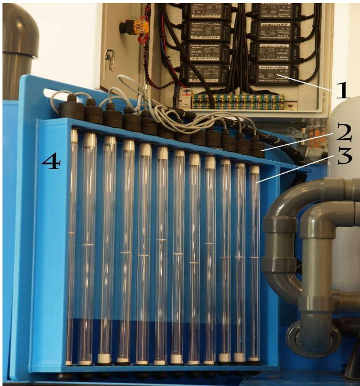
Abb. 2: 12 x UV-C Lampe mit jeweils 20 W
